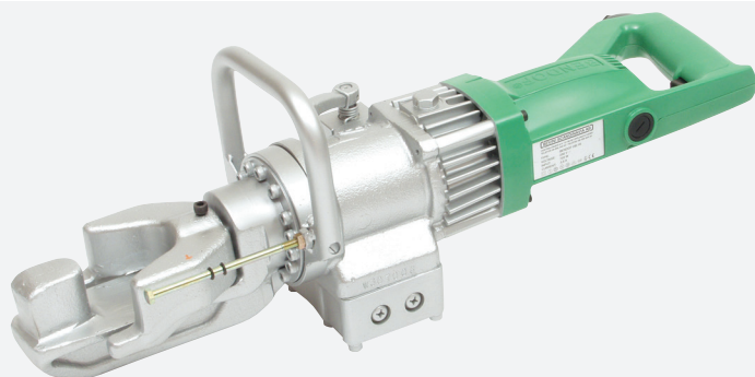
Håndholdt armeringsbøyemaskin 720W HB-16
